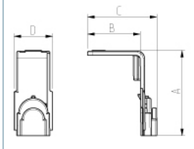
Rysunek przekrojowy 2
