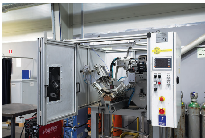
Automatyczna spawarka korpusów szafek SWN
